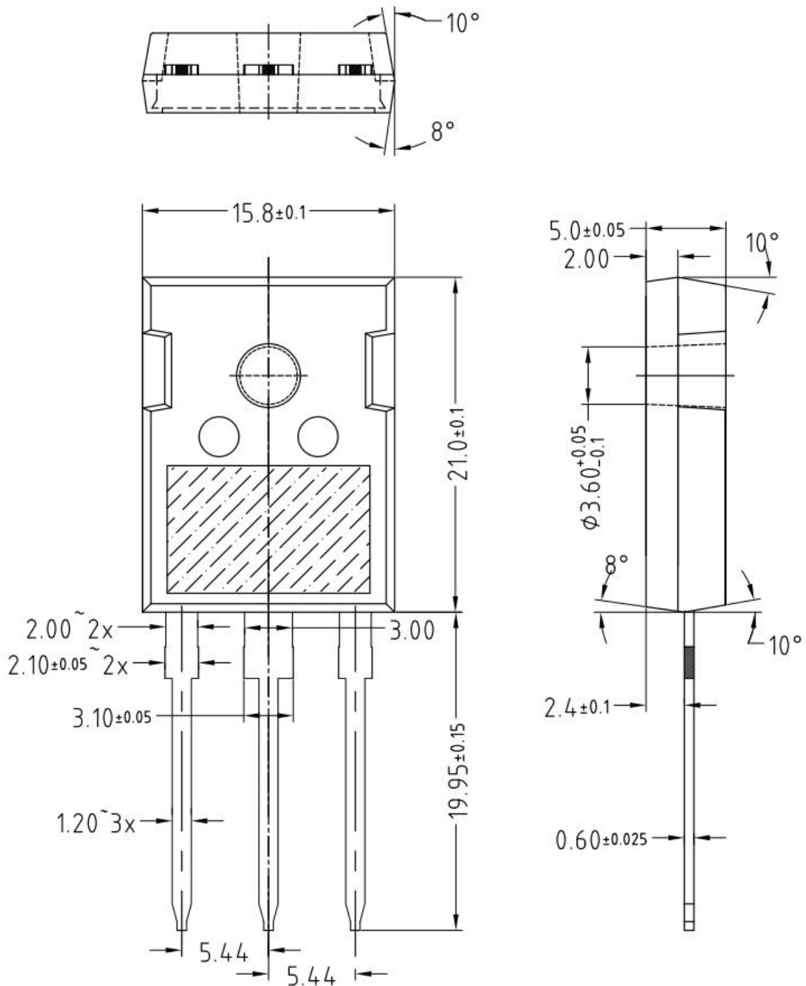
TO-247-3L
